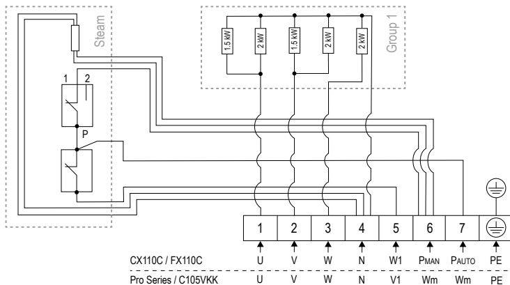
Abbildung 5. Stromlaufplan CR100S
