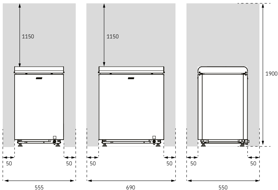
Рисунок 1. Безопасное расстояние
