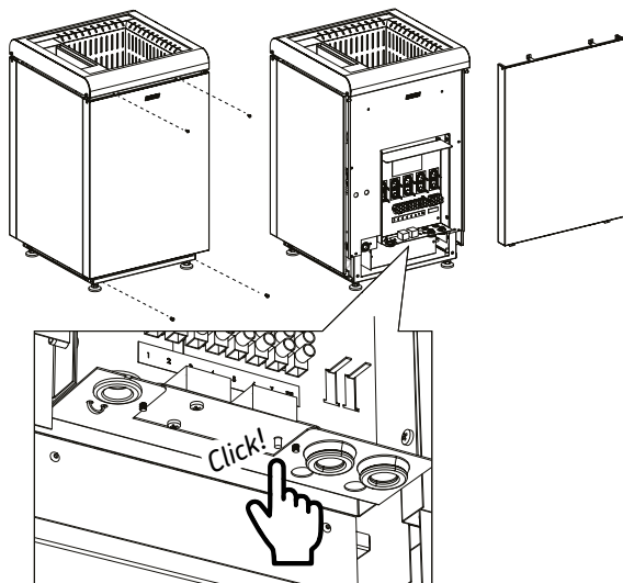
Figure 13. Réinitialisation de la sécurité-surchauffe de l'évaporateur
