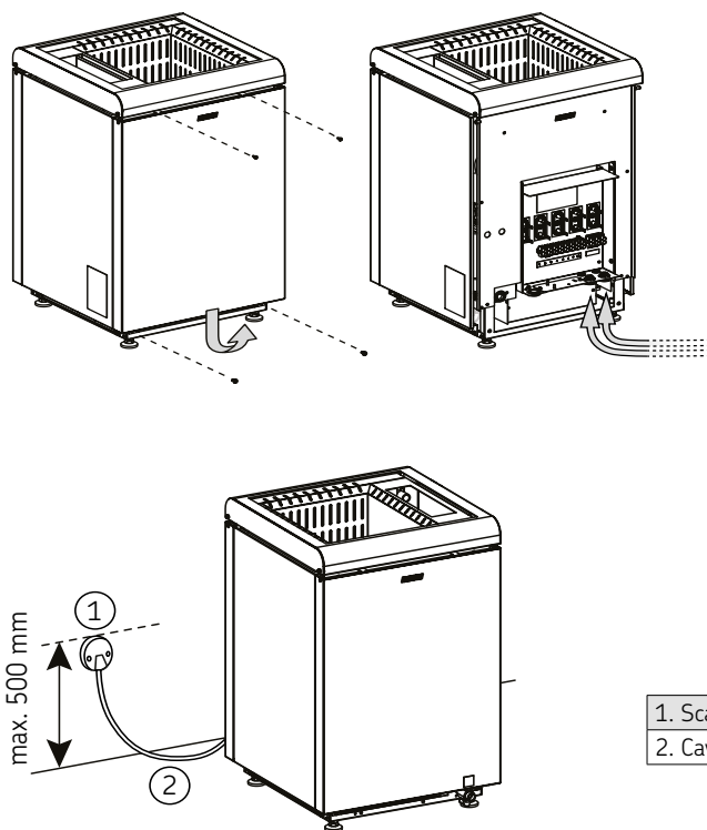
Figura 4. Collegamenti elettrici
