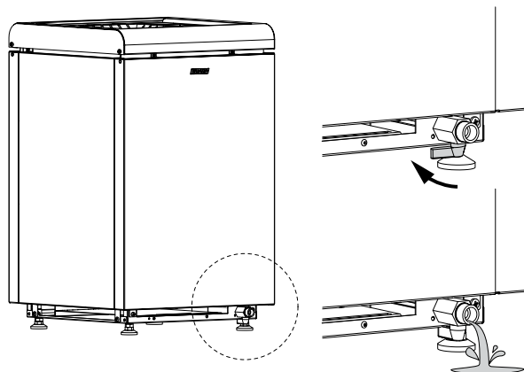
Rysunek 11. Opróżnianie zbiornika na wodę
