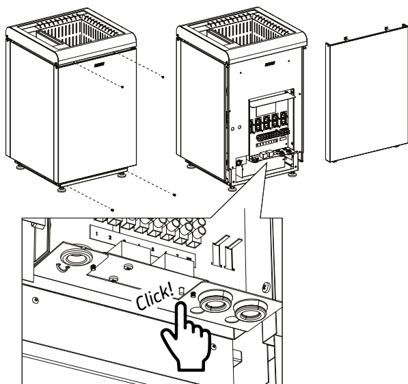
13 pav. Garintuvo apsaugos nuo perkaitimo grįžtis
