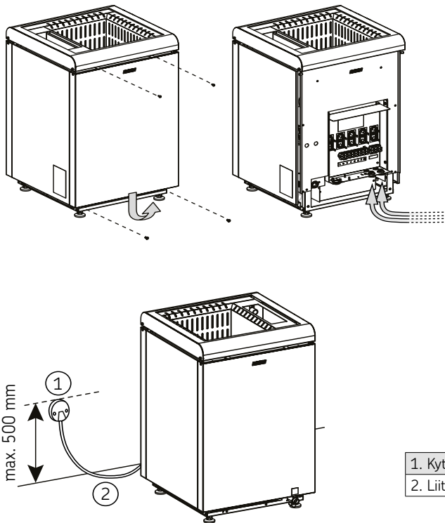
Kuva 4. Sähkökytkennät
