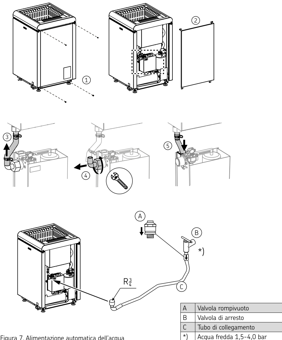
Figura 7. Alimentazione automatica dell'acqua
