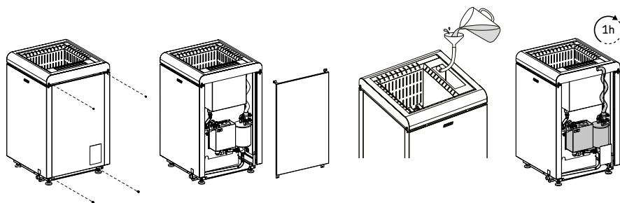
Рисунок 12. Удаление накипи раствором лимонной кислоты
