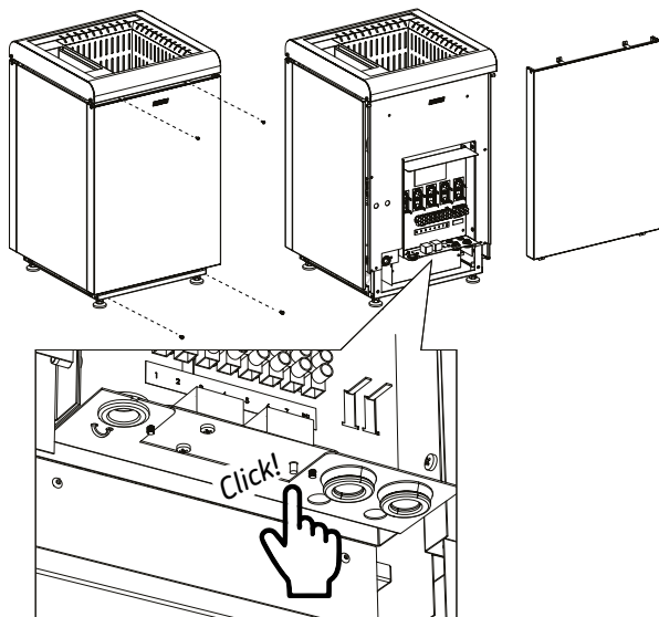
Kuva 13. Höyrystimen ylikuumenemissuojan kuittaus
