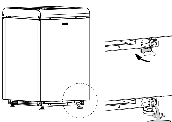
Joonis 11. Veepaagi tühjendamine
