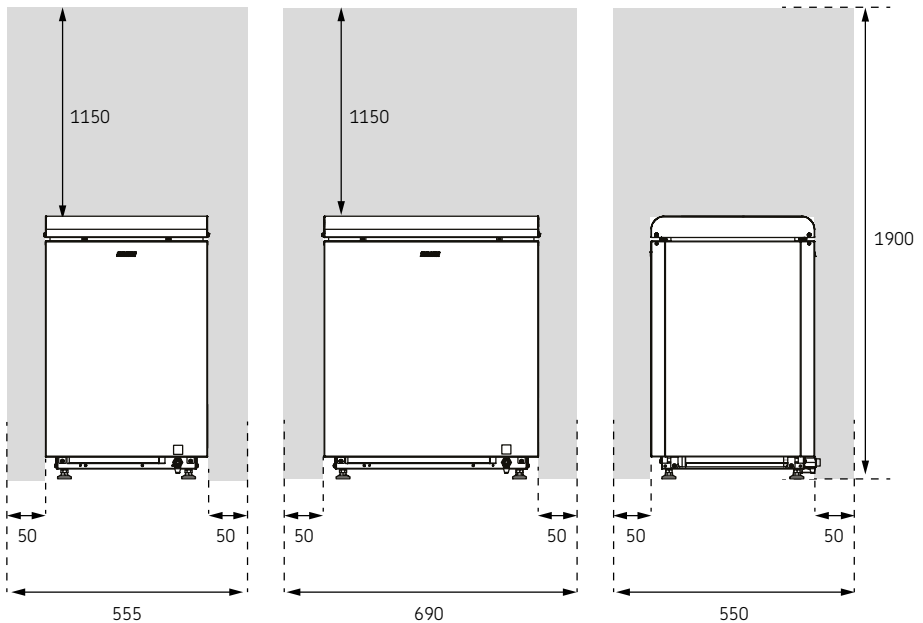
Abbildung 1. Sicherheitsabstände
