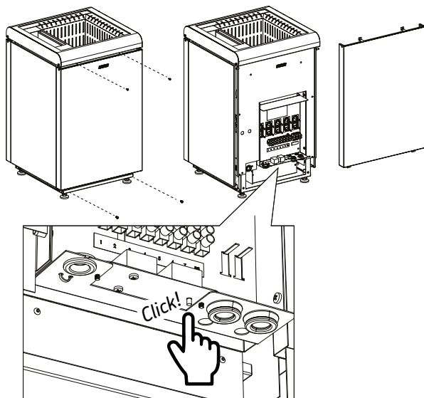
Figuur 13. Reset de beveiliging tegen oververhitting van de stoomgenerator
