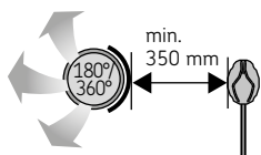
Bild 9. Minimiavstånd mellan tilluftsventil och temperaturgivare.
