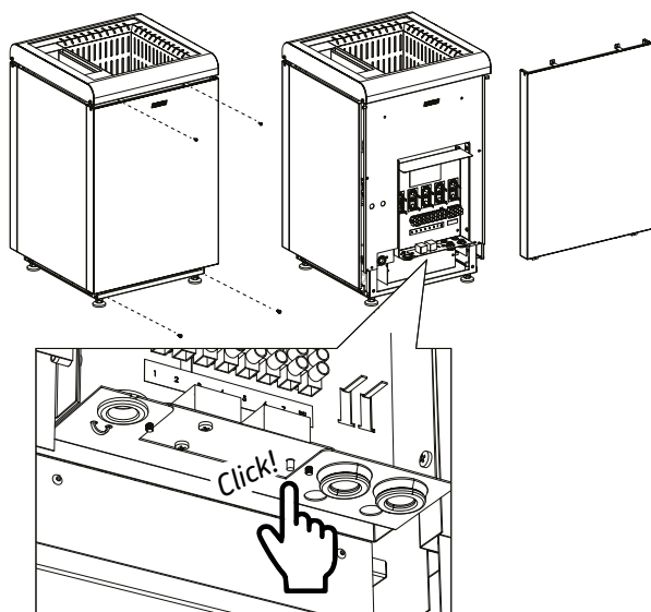
Obrázek 13 Resetování ochrany proti přehřátí parního generátoru
