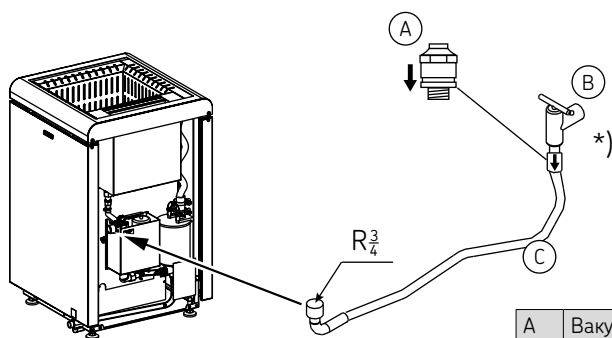
Рисунок 7. Автоматическая подача воды
