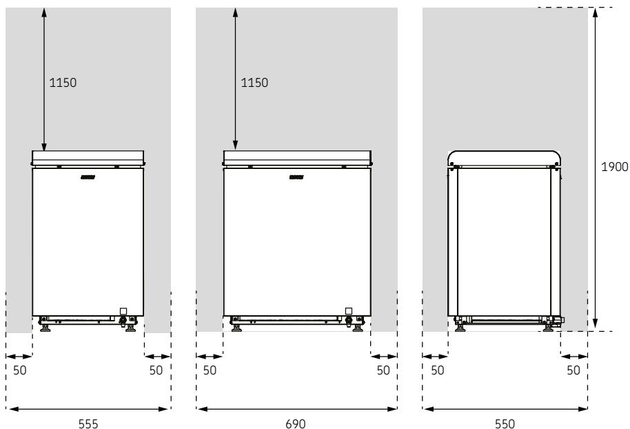
Obrázek 1 Bezpečnostní vzdálenosti
