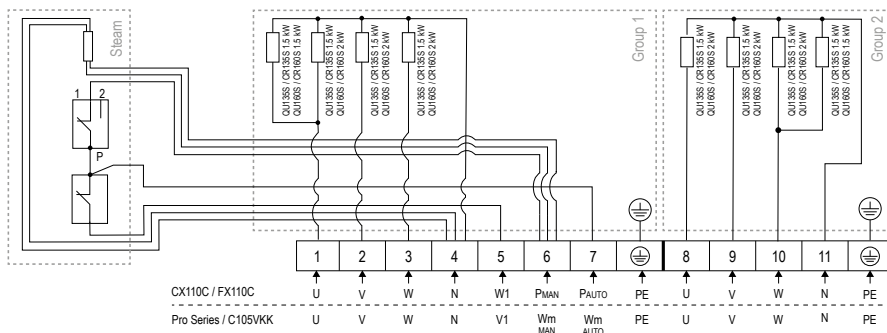
Abbildung 6. Stromlaufplan CR135S, CR160S
