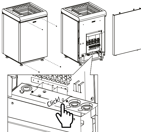
Abbildung 13. Zurücksetzen des Überhitzungsschutzes des Verdampfers
