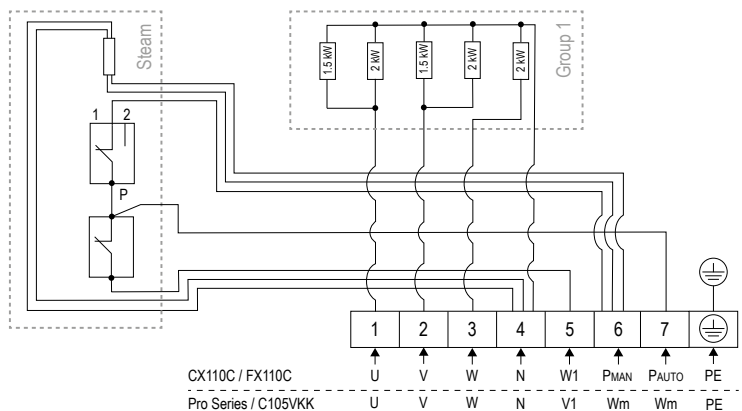
Kuva 5. Kytentäkaavio CR100S
