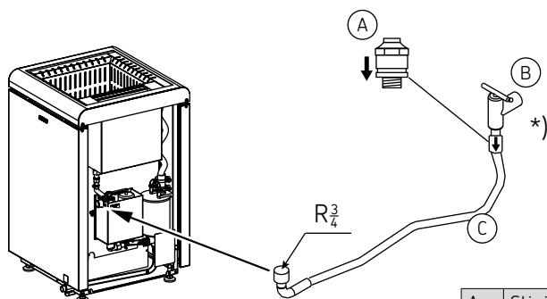
7 pav. Automatinis vandens tiekimas
