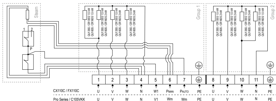
Joonis 6. Elektriskeem CR135S, CR160S
