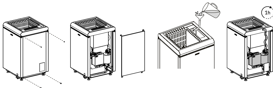
Figura 12. Rimozione del calcare con una soluzione di acido citrico
