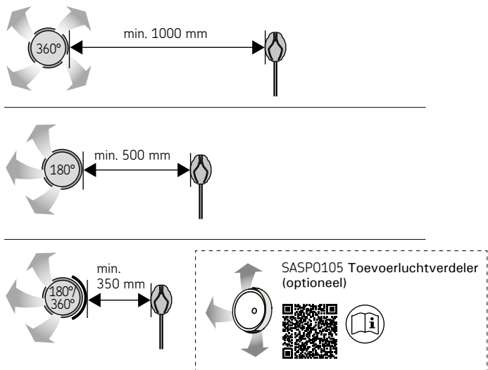
Figuur 9. Minimale afstand van de luchttoevoerklap tot de temperatuursensor.
