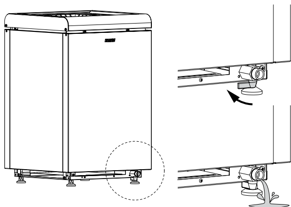
Figuur 11. De watertank legen
