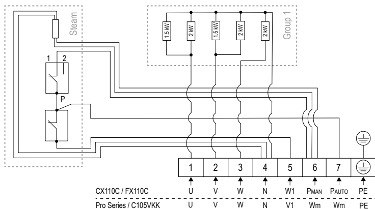
Figure 5. Schéma de câblage CR100S
