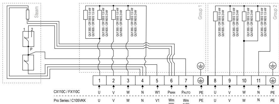
Bild 6. Kopplingsschema CR135S, CR160S
