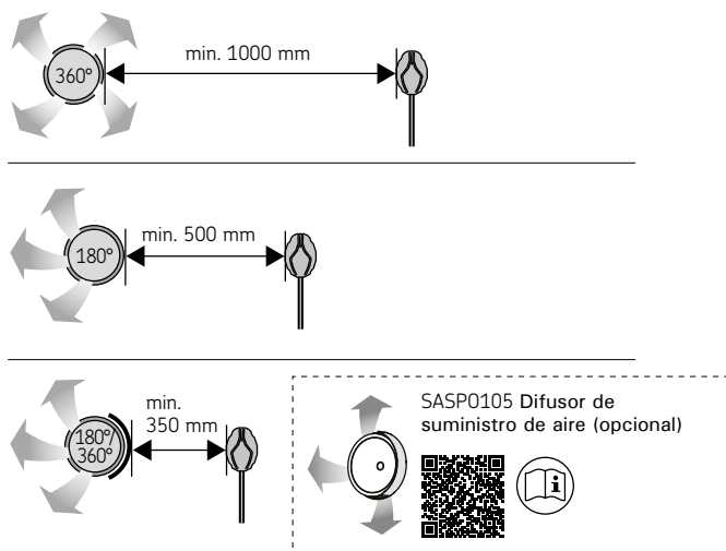
Figura 9. Distancia mínima entre la salida de suministro de aire y el sensor de temperatura.
