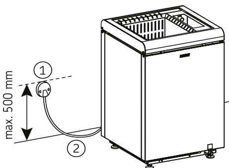
Rysunek 4. Połączenia elektryczne
