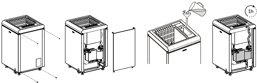
Kuva 12. Kalkinpoisto sitruunahappoliuoksella
