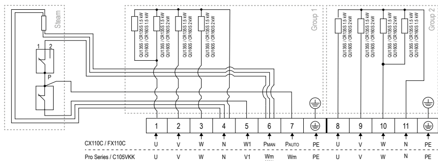
Figura 6. Esquema eléctrico CR135S, CR160S
