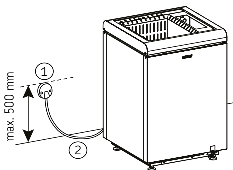
Рисунок 4. Электрические соединения
