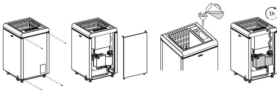
Figure 12. Détartrage avec une solution d'acide citrique
