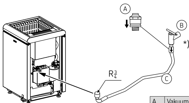
7. attēls. Automātiskā ūdens padeve
