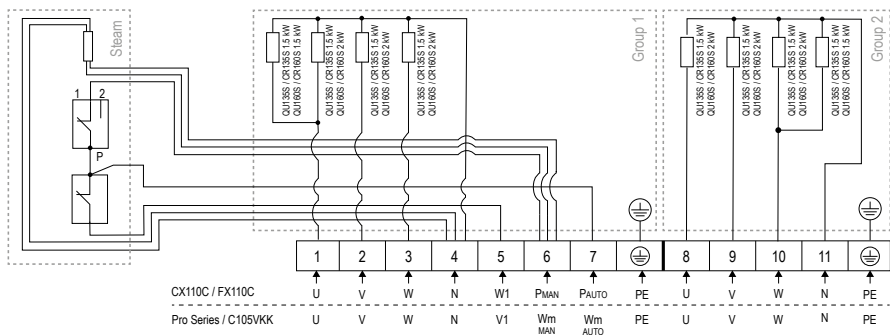
Obrázek 6 Schéma zapojení CR135S, CR160S
