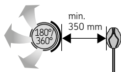
Obrázek 9 Minimální vzdálenost od větracího otvoru přívodu vzduchu k teplotnímu senzor
