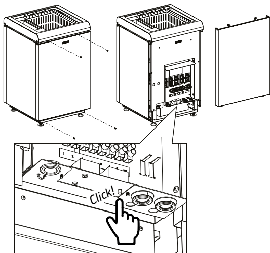
Figura 13. Ripristino della protezione termica di sicurezza dell'umidificatore
