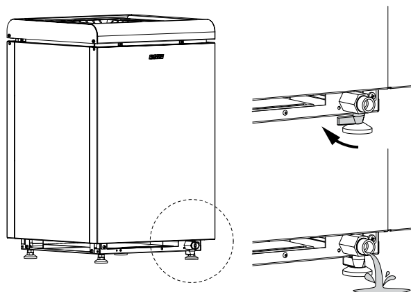
Obrázek 11 Vyprázdnění nádržky na vodu
