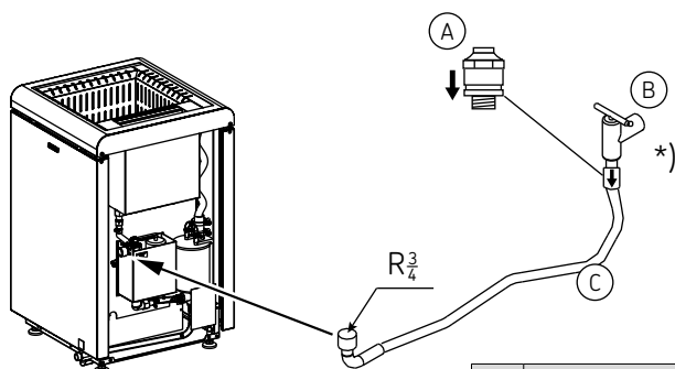
Figure 7. Alimentation automatique en eau
