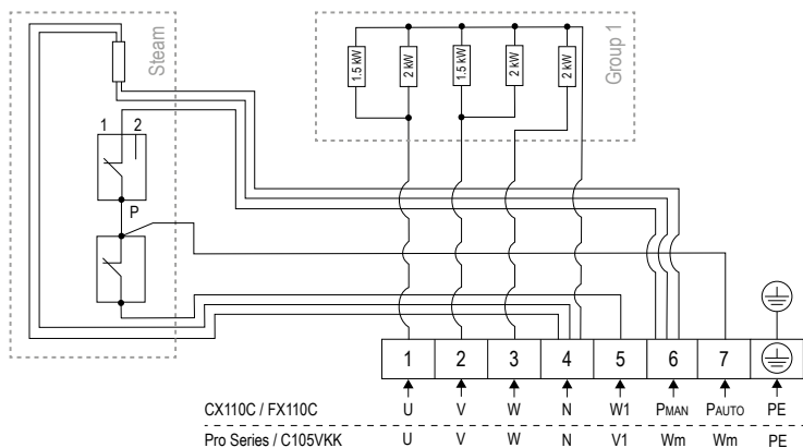
Slika 5. Shema ožičenja CR100S
