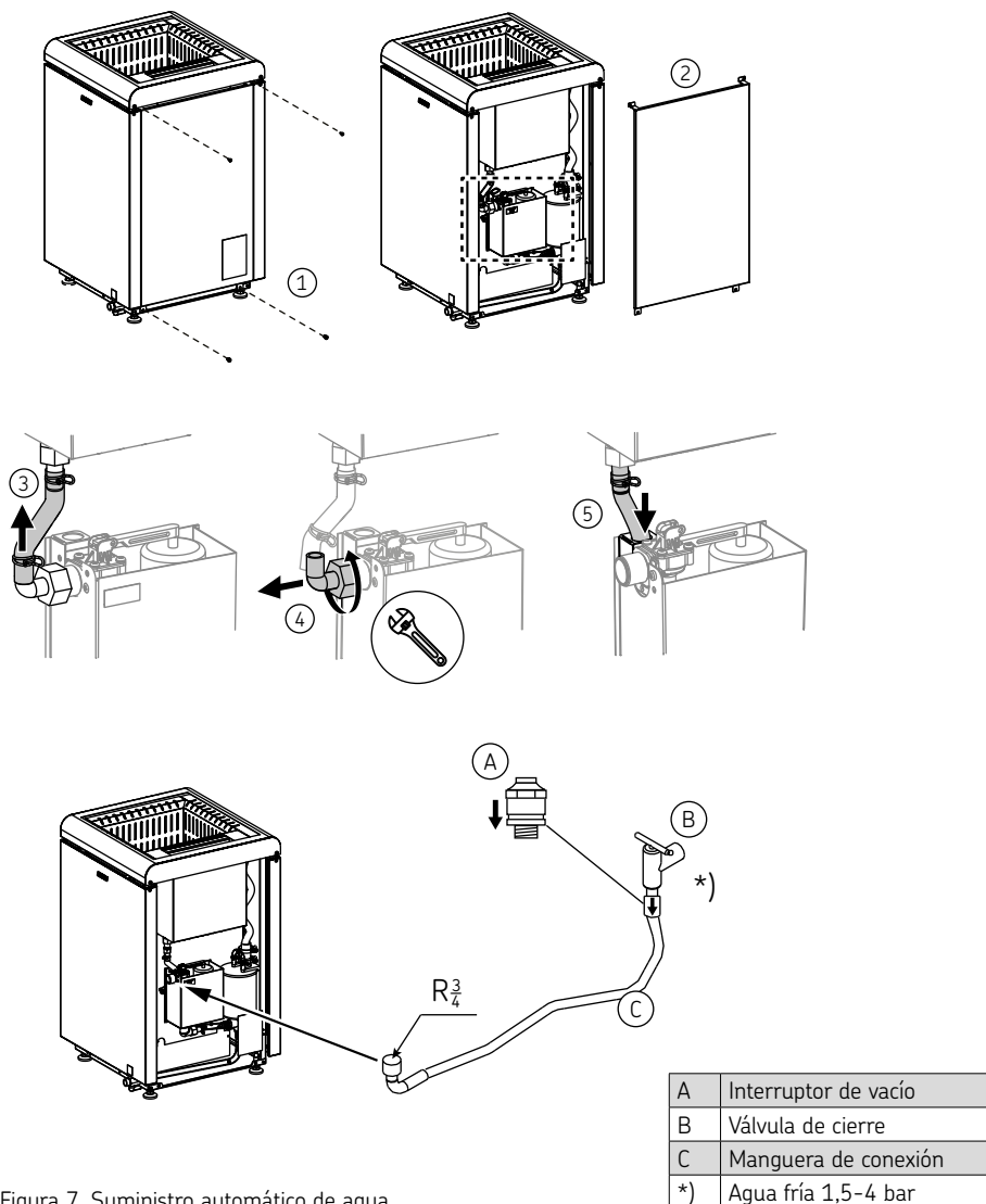
Figura 7. Suministro automático de agua
