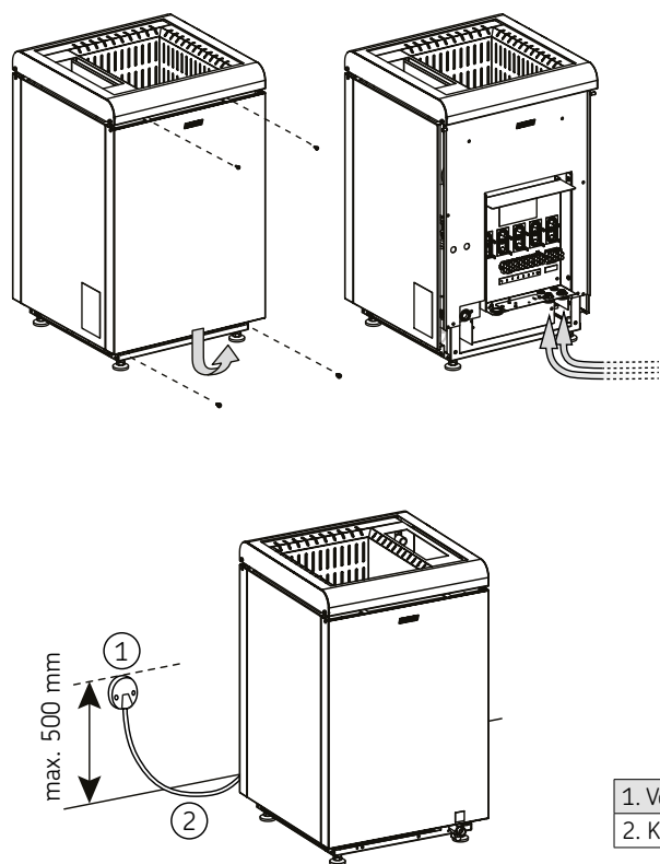
Abbildung 4. Elektroanschlüsse
