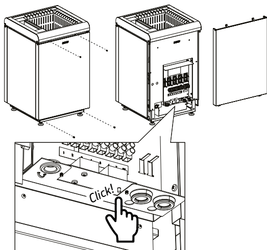
Figura 13. Reinicio del seguro de recalentamiento del vaporizador
