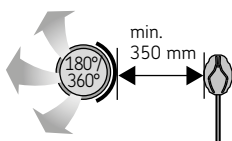
Abbildung 9. Mindestabstand des Fühlers zur Luftzufuhr.
