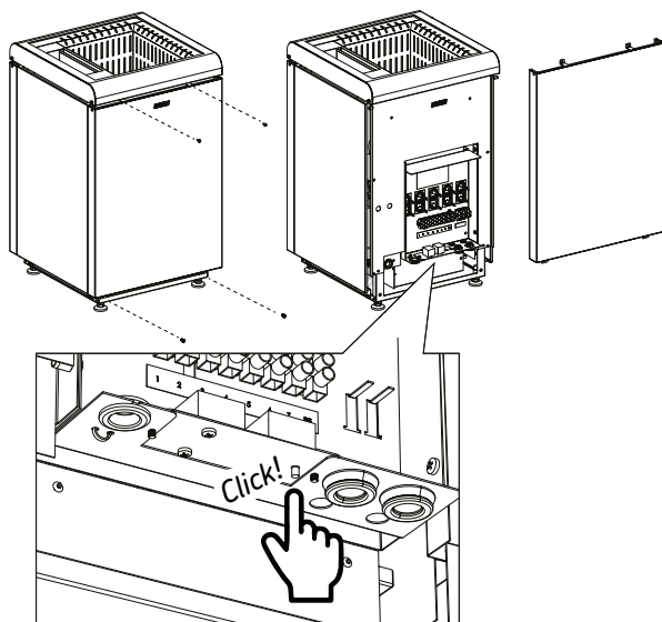
Рисунок 13. Сброс защиты от перегрева в парогенераторе
