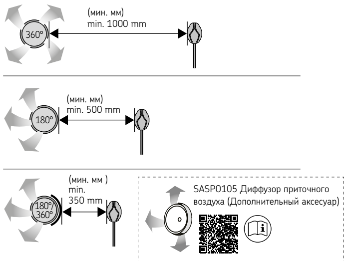
Рисунок 9. Минимальное расстояние от температурного датчика до вентиляционной отдушины.
