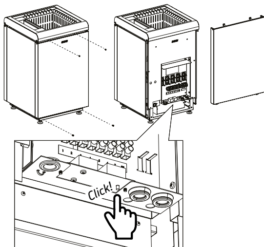
Rysunek 13. Resetowanie bezpiecznika termicznego parownika
