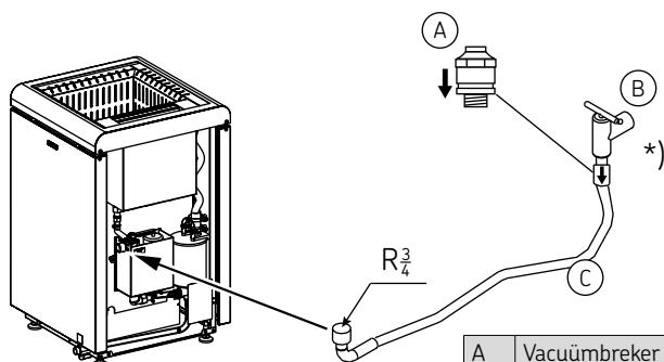
Figuur 7. Automatische watertoevoer
