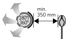
Figura 9. Distanza minima tra lo sfiato dell'aria di alimentazione e il sensore di temperatura.
