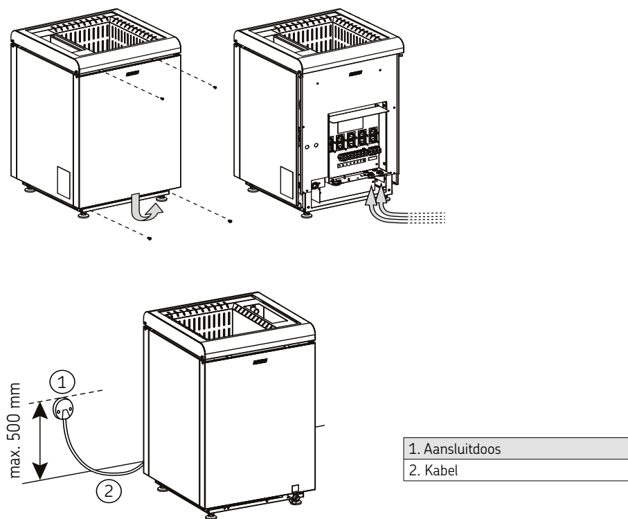
Figuur 4. Elektrische aansluitingen
